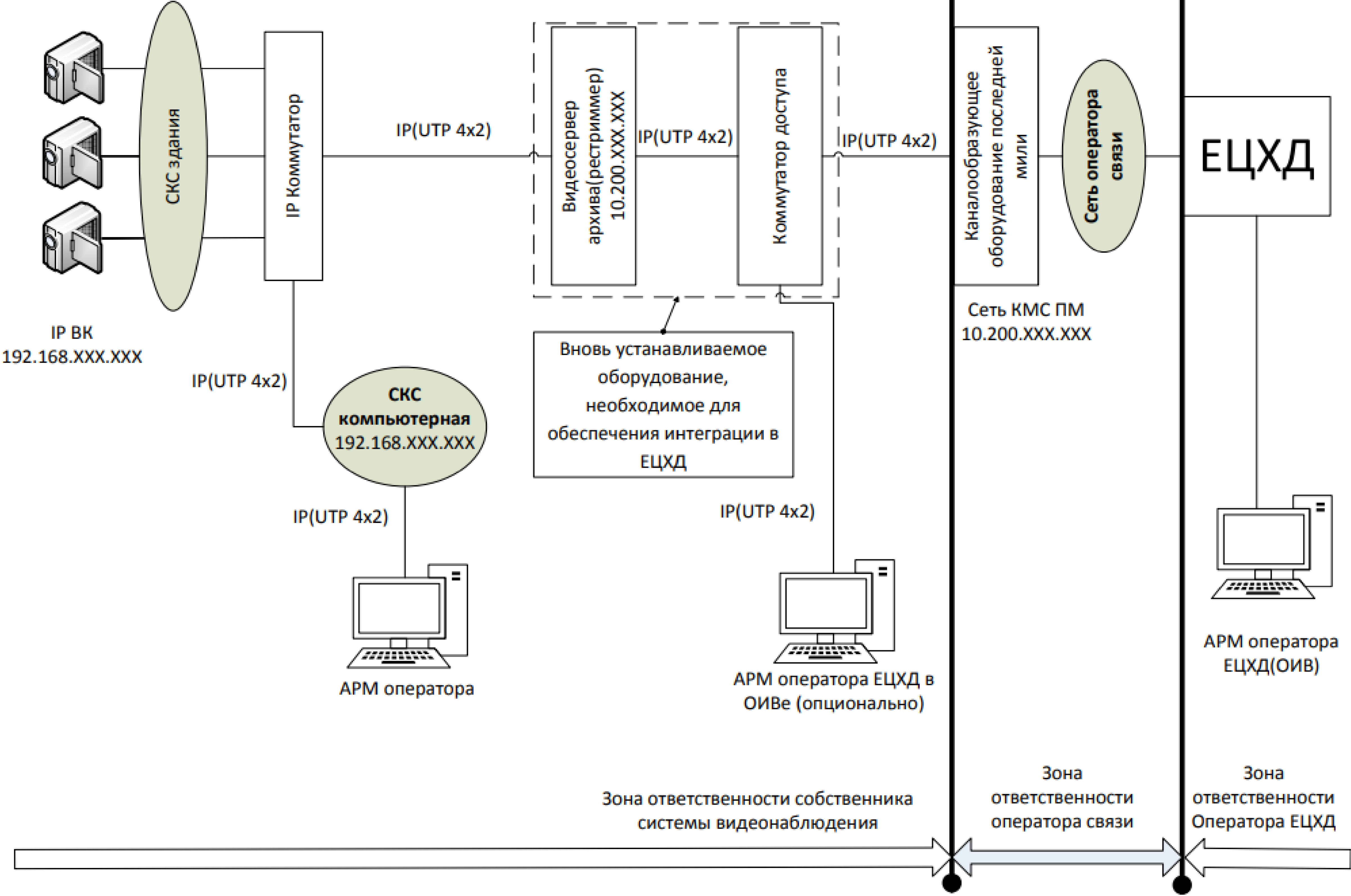
Схема интеграции внешней системы IP видеонаблюдения в ЕЦХД
